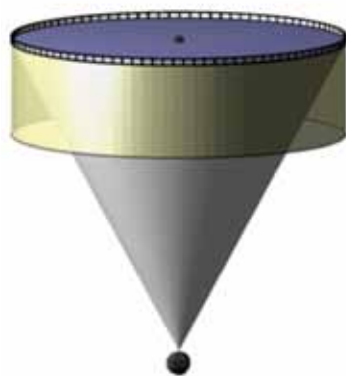
Figur 7.1-1. Venstre: Prinsippet bak presenningskjørt eller planktondukskjørt rundt de øvre metrene av en merd. Høyre: Figur av målt vannstrøm i og rundt en standard merd med et 5 m dypt tilpasset presenningskjørt [148]. (Illustrasjoner Lars H. Stien.)
