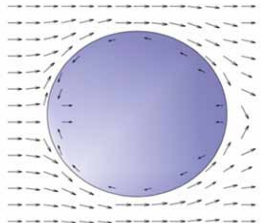
Figur 7.1-1. Venstre: Prinsippet bak presenningskjørt eller planktondukskjørt rundt de øvre metrene av en merd. Høyre: Figur av målt vannstrøm i og rundt en standard merd med et 5 m dypt tilpasset presenningskjørt [148]. (Illustrasjoner Lars H. Stien.)
