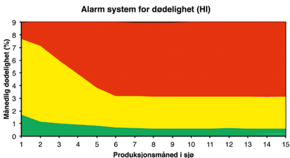
Figur 3.5-1. Standard dødelighetskurve for de første 15 måneder etter sjø utsett [80], er basert på data som rapporteres av den norske lakseindustrien fra 2009 til 2015 til Fiskeridirektoratet (på månedlig basis). 75 % av alle observasjonene er i det grønne området og kan kategoriseres som «normale», mens 5 % av observasjonene er i det røde området og er kategorisert som «unormale», dvs. med økt dødelighet. (Lars H. Stien, ikke publiserte data.)
