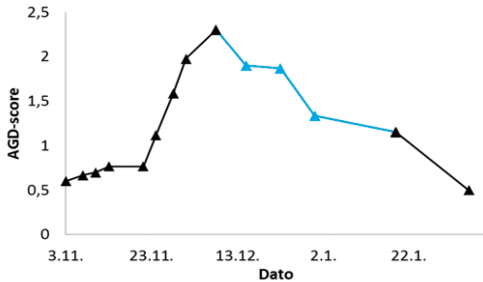
Figur 5.7.-1. Gjennomsnittlig AGD gjelleskår registrert med ukentlig basis hos oppdrettere basert på en 5-punkts AGD-skala. Blå symbol og linje indikerer perioden hvor ferskvann ble tilført snorkelen. (Lars H. Stien ikke publiserte data.)
