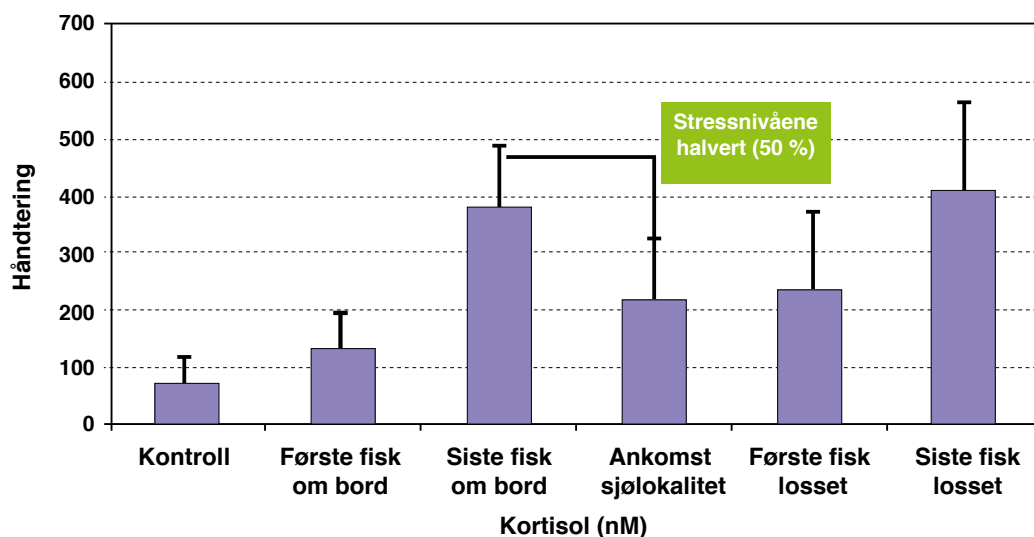
Figur 1.8-2. Gjennomsnittlig plasmakortisol før, under og etter brønnbåttransport. Legg merke til hvordan plasmakortisol er redusert med ca. 50 % etter ankomst i sjøen, noe som gir laksen god gjenvinning av normale livsfunksjoner mellom de to store stressorene lasting og lossing. Figur hentet fra Iversen og Eliassen [125]. Gjengitt med tillatelse fra M.H. Iversen.
