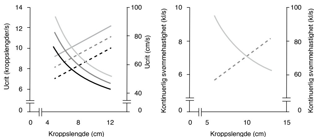
Figur 4.2.1-1. A) Den kritiske relative (kroppslengder/s, heltrukne linjer) og absolutte (cm/s, stiplede linjer) svømmehastigheten av atlantisk lakseparr som en funksjon av fiskelengden ved 12 °C (lys grå), 16 °C (mørk grå) og 20 °C (svart). Data fra Peake mfl. (1997). B) Maksimal kontinuerlig svømmehastighet hos parr som en funksjon av kroppslengde i temperaturområdet 12,5 til 19 °C. Heltrukket linje indikerer relativ hastighet (kroppslengder/s) og stiplet linje absolutt hastighet (cm/s). Data fra Peake mfl. (1997).
