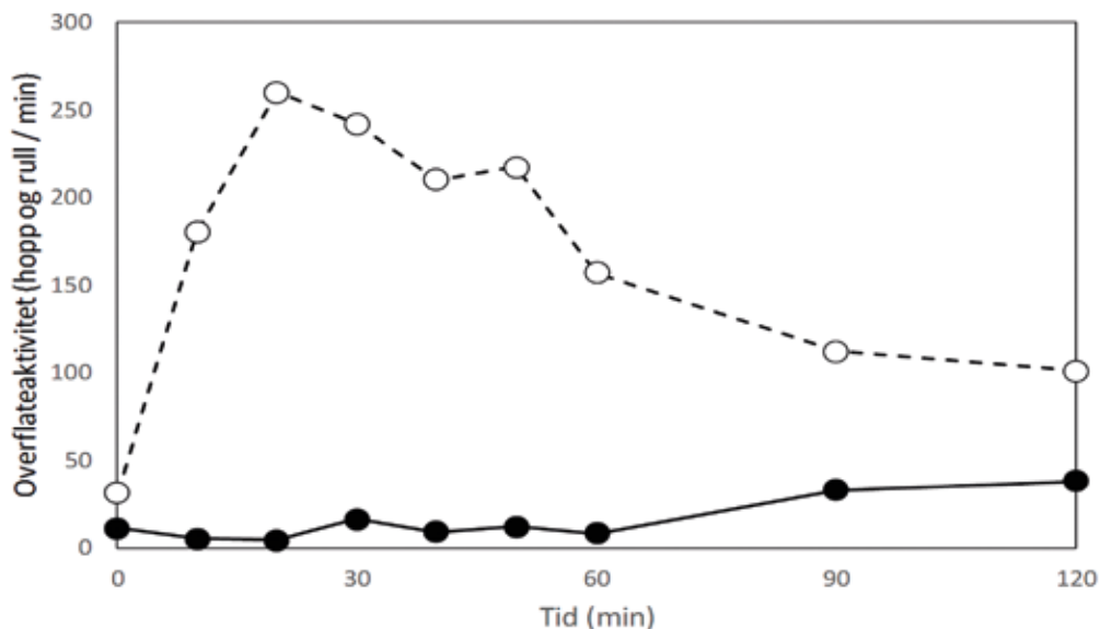
Figur 4.7-2. Overflateaktivitet ved retur til overflaten etter tre ukers neddykking. I det første tilfellet (fylte sirkler med heltrukket linje) har laksen benyttet luftlommen til å fylle svømmeblæren, mens i den andre merden har dette bare vært delvis vellykket og laksen har en sterk trang til å fylle svømmeblæren etter heving (åpne sirkler med stiplet linje). (Lars H. Stien ikke publiserte data.)
