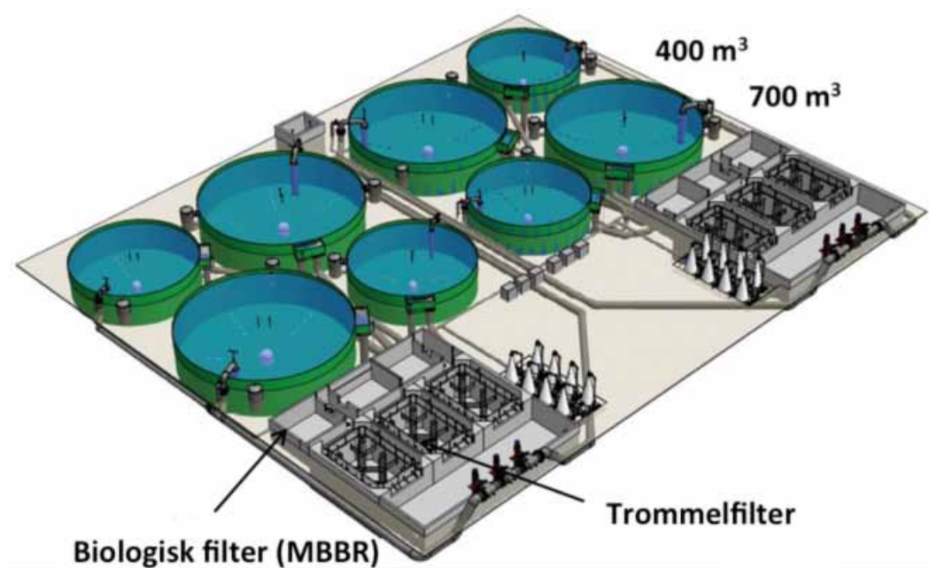
Figur 2.1-1. Skjematisk oversikt over Grieg Seafood kommersielle RAS-anlegg på Adamselv med bevegelige biofilter (mbbs), trommelfiltre, oksygenering og to karstørrelser, 400 og 700 m 3 (Tegning: Frode Mathisen, gjengitt med tillatelse).
