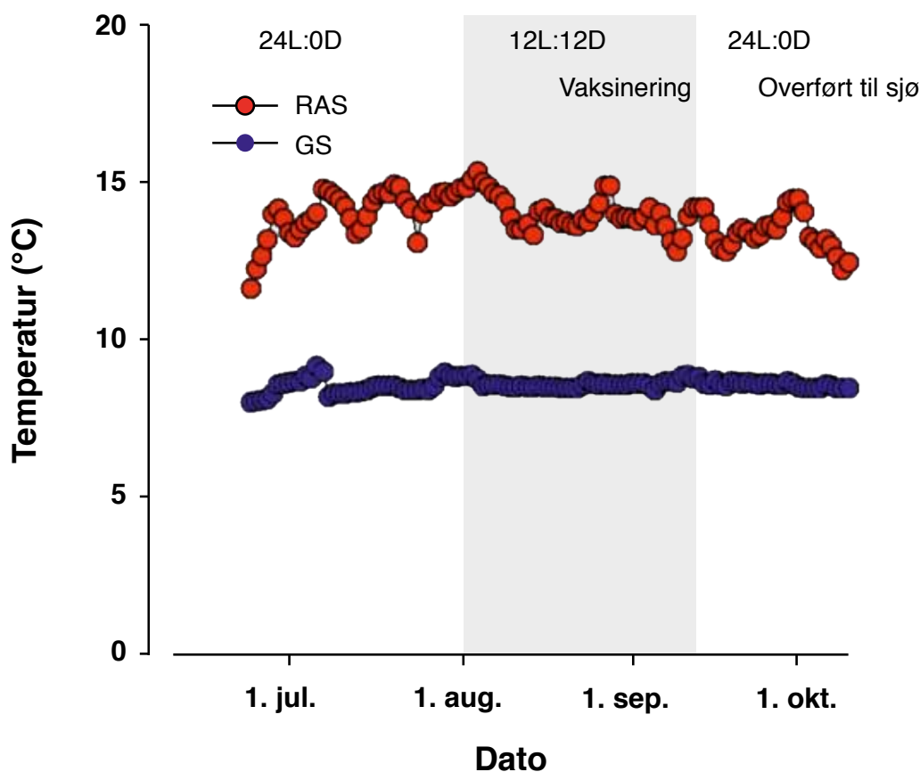
Figur 2.4-1. Eksempel på en temperaturprofil i RAS sammenlignet med et GS-system, hvor RAS-råvann kommer fra den samme kilden som det brukte vannet i GS-systemet. Ingen ekstra oppvarming av RAS-vann ble gjort [59]. (Gjengitt med tillatelse fra J. Kolarevic)
