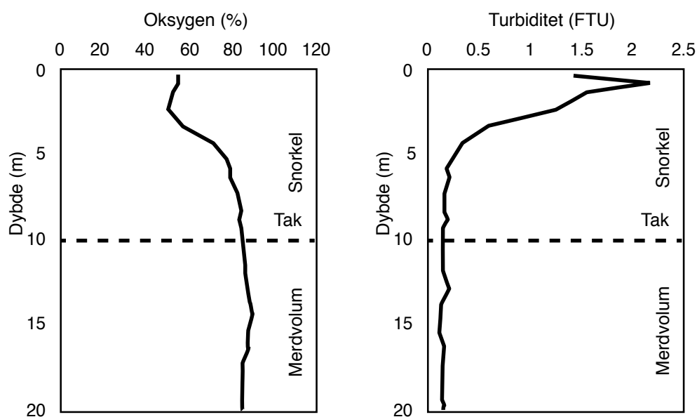
Figur 5.2-1. Oksygen og turbiditet målt i en kommersiell 10 m dyp snorkel, og i merden under. Legg merke til nedgangen i oksygen i toppen av snorkelen og økningen i turbiditet. (Lars H. Stien, ikke publiserte data.)
