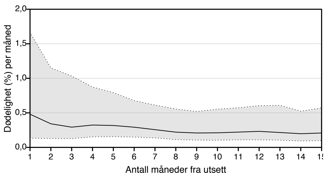
Figur 3.1.1-1. Standard dødelighetskurve for de 15 første månedene i sjø basert på innrapporterte data fra alle norske lakseoppdrettere fra 2009-2015. Kurven gir median månedlig dødelighet, omgitt av 25- og 75-prosentiler.
