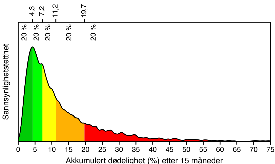
Figur 3.1.1-2. Fordelingen av dødeligheten etter 15 måneder i sjø. 0 til 4,3 % (mørk grønn, bedre enn vanlig velferd), 4,3 til 7,2 % (grønn), 7,2 til 11,2 % (gul), 11,2 til 19,7 % (oransje), > 19,7 % (rød, verre enn vanlig velferd).
