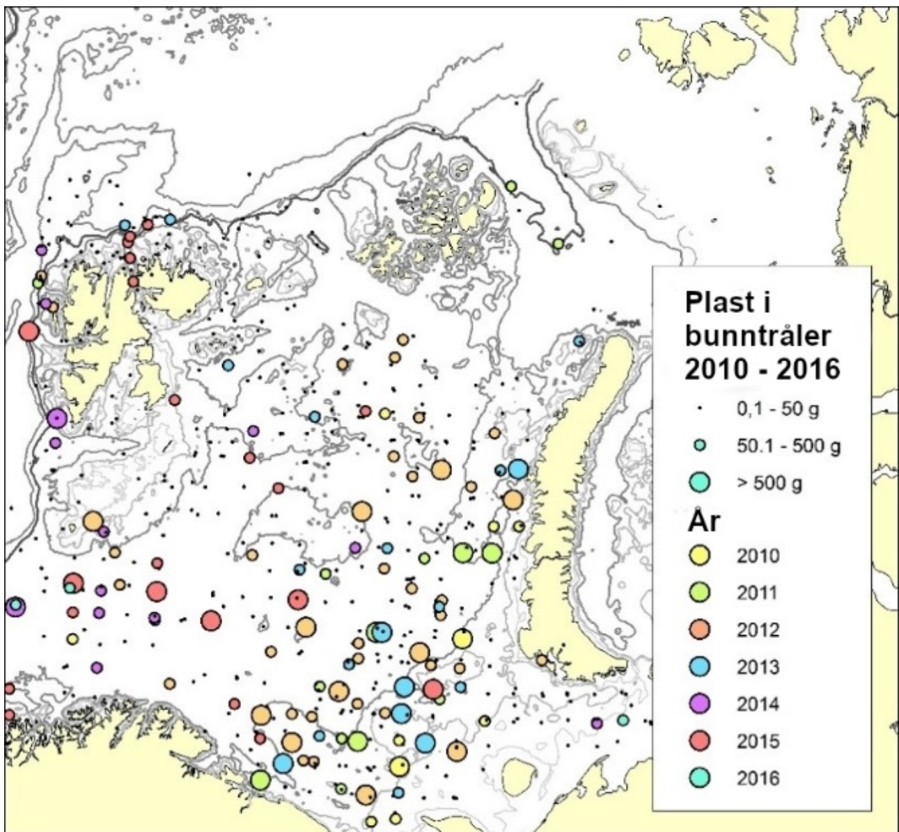
Figur 3.5. Registrering av plast i bunntrawl fra det norsk-russiske økosystemtøktet fra Barentshavet i perioden 2010 til 2016. Ulike farger indikerer ulike år (Grøsvik et al., 2018).
