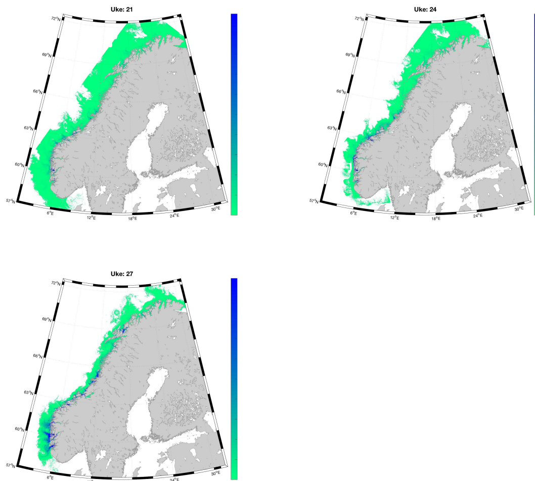
Figur 59. Modellert tetthet av lakseluskopepoditter langs Norskekysten i uke 21, 24 og 27 i 2019. Grønn farge angir lav tetthet og blå farge angir høy tetthet.
