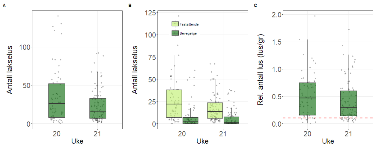
Figur 22. Antall lakselus (A), antall lakselus fordelt på fastsittende og bevegelige stadier (B) og relativt antall lus (antall lus/gram kroppsvekt) (C) fra sjørret fanget i lakserusen ved Måløy.
