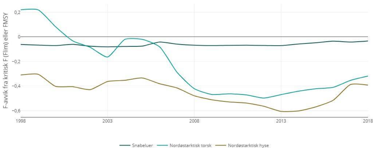
Figur 4.37. Fiskedødelighet for NØA torsk, NØA hyse og snabeluer. Fisket regnes som bærekraftig så lenge F er negativ i forhold til vedtatt fiskedødelighetsgrense (0). Dataene er hentet fra beregningene fra det internasjonale havforskerrådet ICES (ICES 2020).
