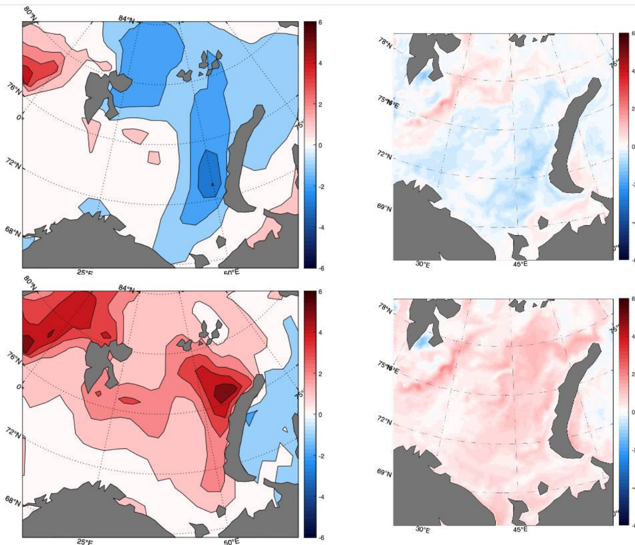
Figur 4.13. Forventede endringer i atmosfæretemperatur fra NorESM ( ^{\circ}\text{C} , venstre) og overflatetemperatur i havet fra ROMS ( ^{\circ}\text{C} , høyre) for mars fra årene 2010-2019 til henholdsvis 2026-2035 (øverst) og 2060-2069 (nederst). Blått indikerer nedkjøling og rødt indikerer oppvarming.
