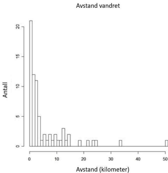
Figur 17. Avstand mellom slippsted og gjenfangststed for torsk merket på Smøla i perioden 2017-2019.
