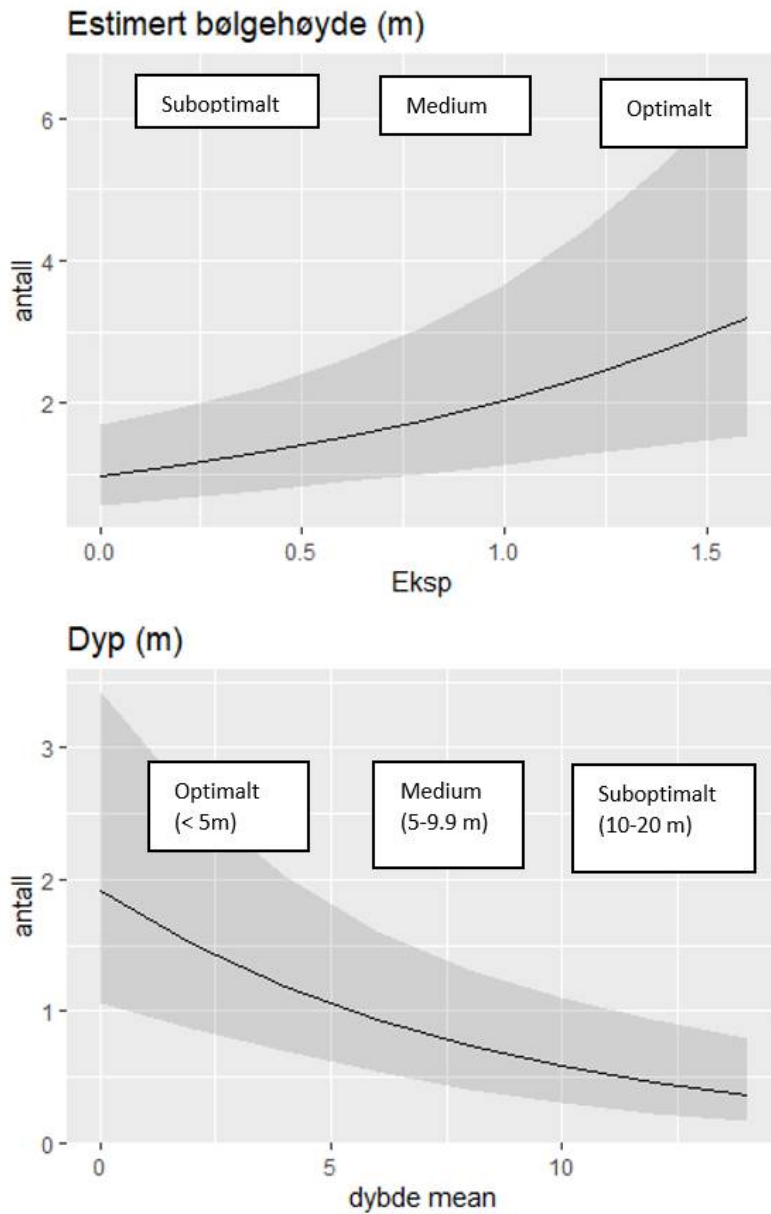
Figur 22. Korrelasjoner mellom estimert fangstrate av berggylt (antall) og bølgeeksponering (øvre diagram) og fangstdyp (nedre diagram). Basert på disse kurvene har vi klassifisert optimalt, medium og sub-optimalt habitat.
