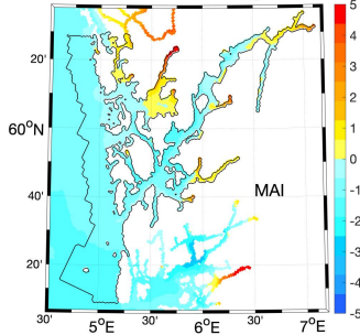
Anomali av overflatesaltholdighet for 2021
