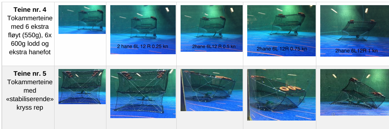
Figur 4. Bilder og beskrivelse av de 5 ulike riggingene av tokammerteinen som ble testet ut i strømtanken under økende strømforhold fra 0 to 1 knop.
