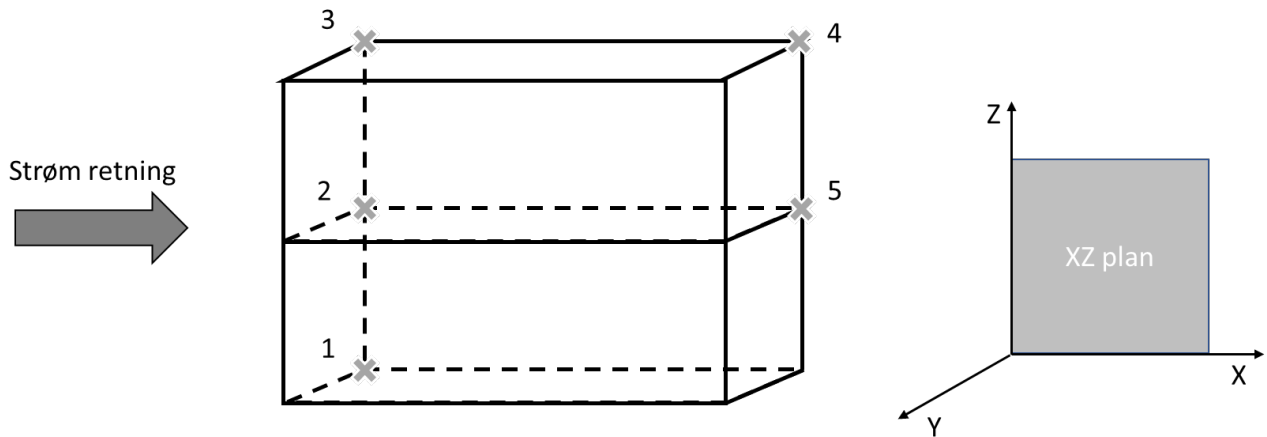
Figur 3. Målingspunkter (1,2,3,4 og 5) for laser markert på teinen.
