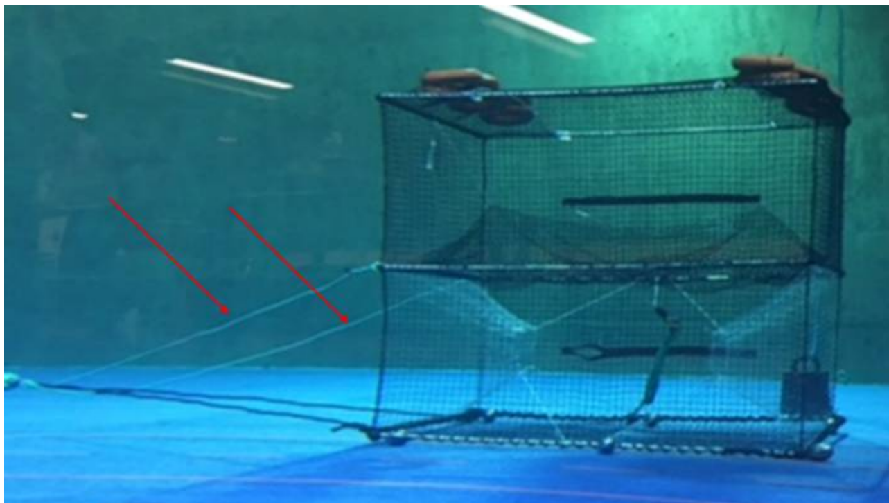
Plassering av ekstra hanefot i midterste ramme.
