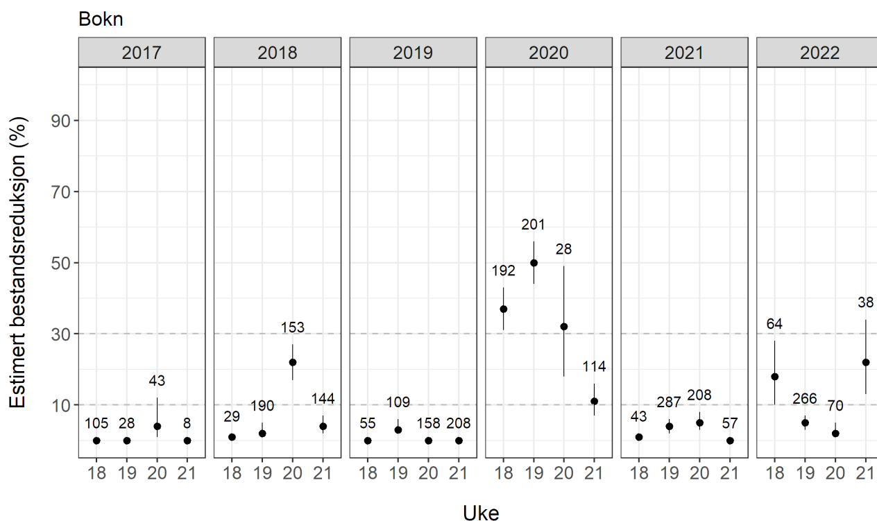
Figur 9. Risiko for lakselusrelatert dødelighet (med konfidensintervaller) som snitt av all trålfanget vill postsmolt av laks fanget hver uke i Boknafjorden. Antall undersøkt hver uke er angitt i figuren.
