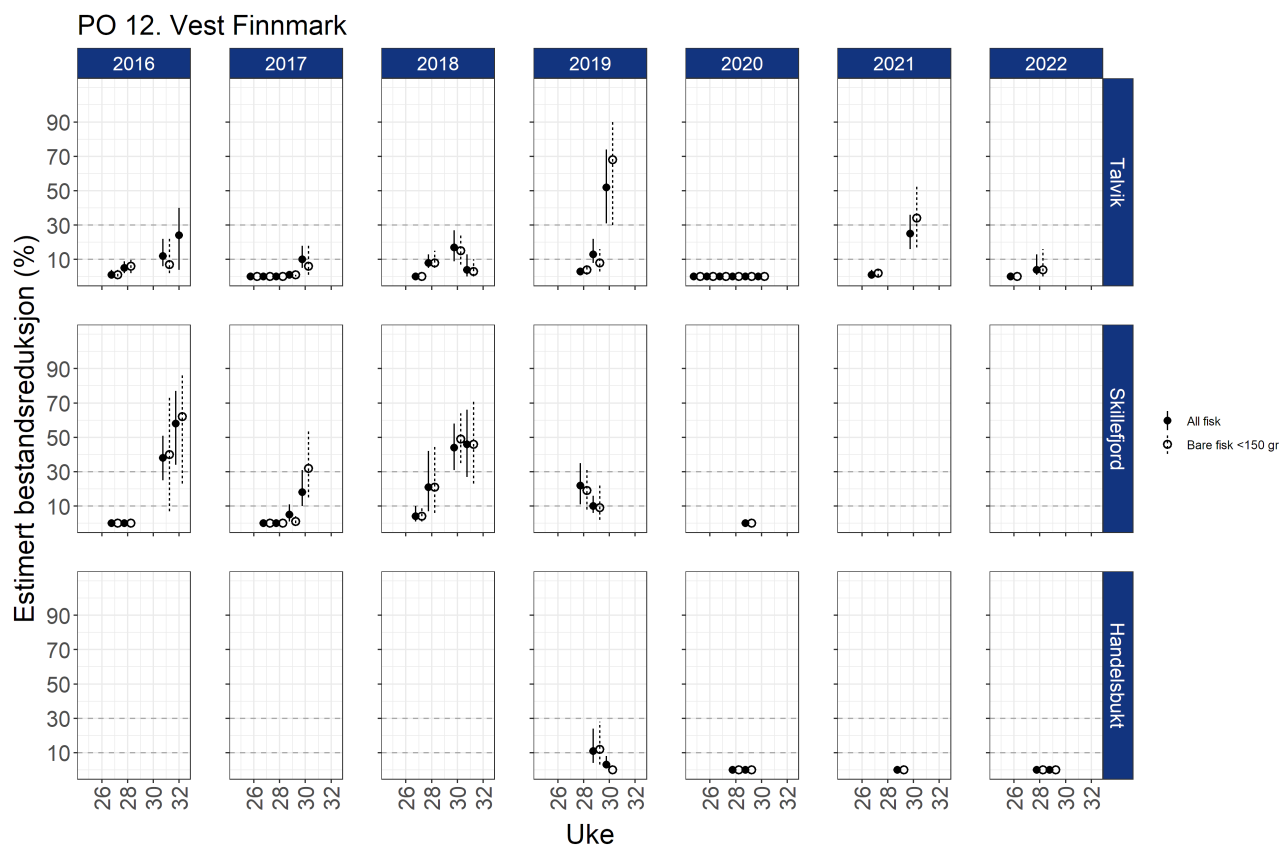
Figur C12: Estimert risiko for dødelighet med konfidensintervaller for sjørret/sjørøye fanget på stasjonene i PO12 beregnet enten ved å bare inkludere fisk < 150 g, eller all sjørret/sjørøye fanget.
