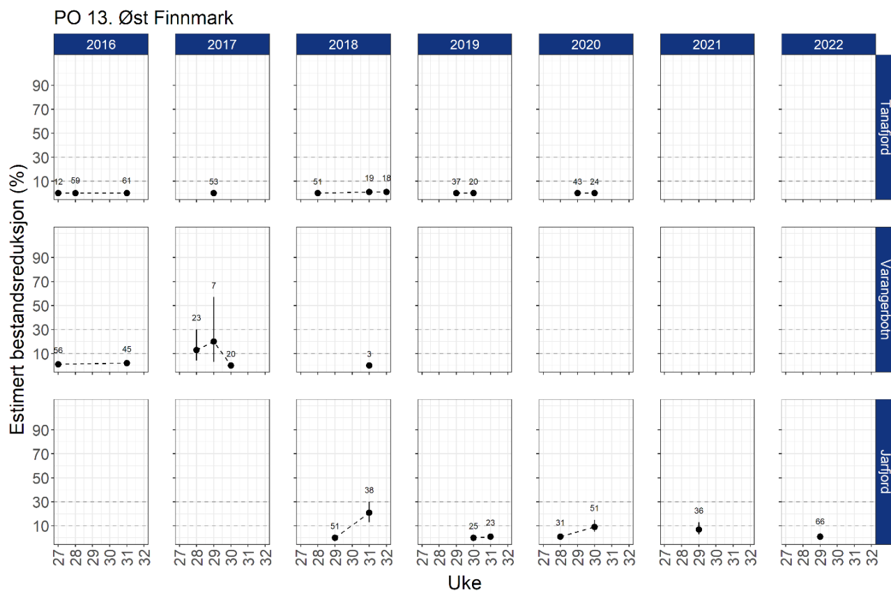
Figur 66. Estimert luseindusert dødelighet på rusefanget sjøørret/sjørøye med 95% konfidensintervaller. Alle beregningene er basert på all fisk fanget og alle lusestadier.
