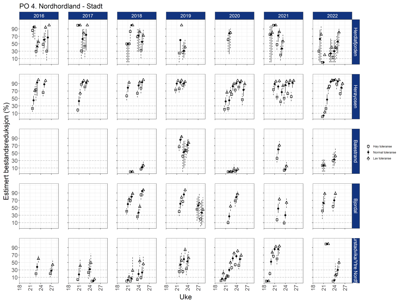
Figur A4. Estimert risiko for dødelighet med konfidensintervaller for sjørøret fanget på stasjonene i PO4 beregnet ved å benytte standard (sirkler), lav (trekanter) eller høy (firkanter) toleransegrenser (Tabell A1). Alle beregningene er basert på sjørøret/sjørøye < 150 g.
