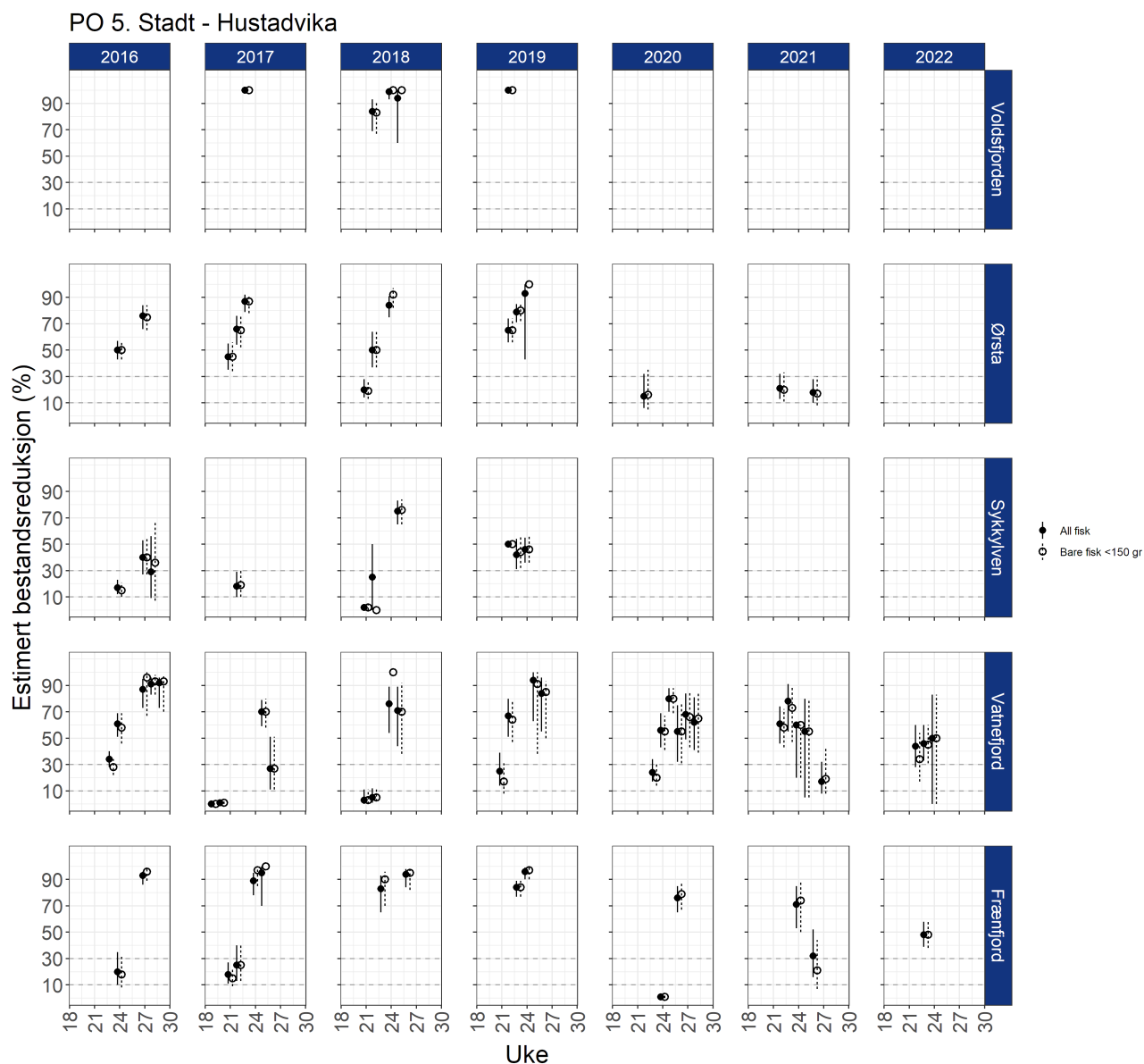
Figur C5: Estimert risiko for dødelighet med konfidensintervaller for sjørøret/sjørøye fanget på stasjonene i PO5 beregnet enten ved å bare inkludere fisk < 150 g, eller all sjørøret/sjørøye fanget.
