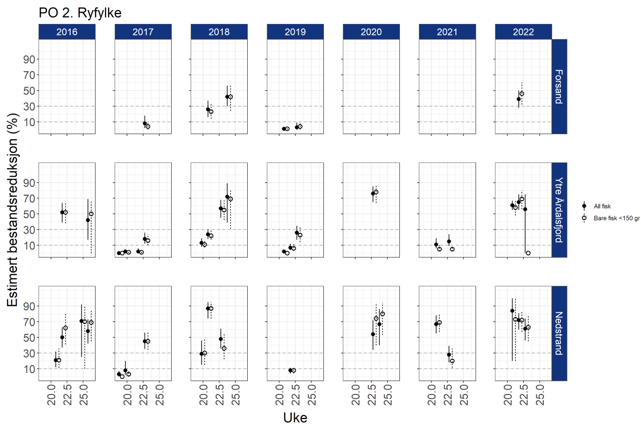
Figur C2: Estimert risiko for dødelighet med konfidensintervaller for sjørret/sjørøye fanget på stasjonene i PO2 beregnet enten å bare inkludere fisk < 150 g, eller all sjørret/sjørøye fanget.
