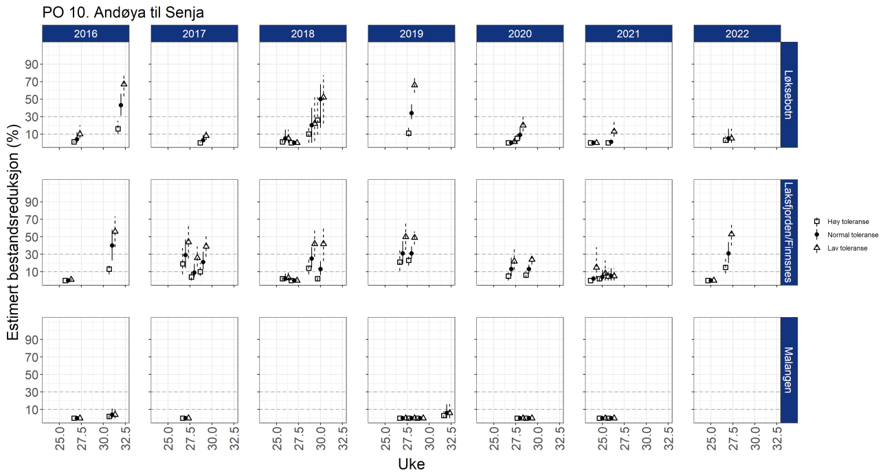
Figur A10. Estimert risiko for dødelighet med konfidensintervaller for sjørøret/sjørøye fanget på stasjonene i PO10 beregnet ved å benytte standard (sirkler), lav (trekanter) eller høy (firkanter) toleransegrenser (Tabell A1). Alle beregningene er basert på sjørøret/sjørøye < 150 g.
