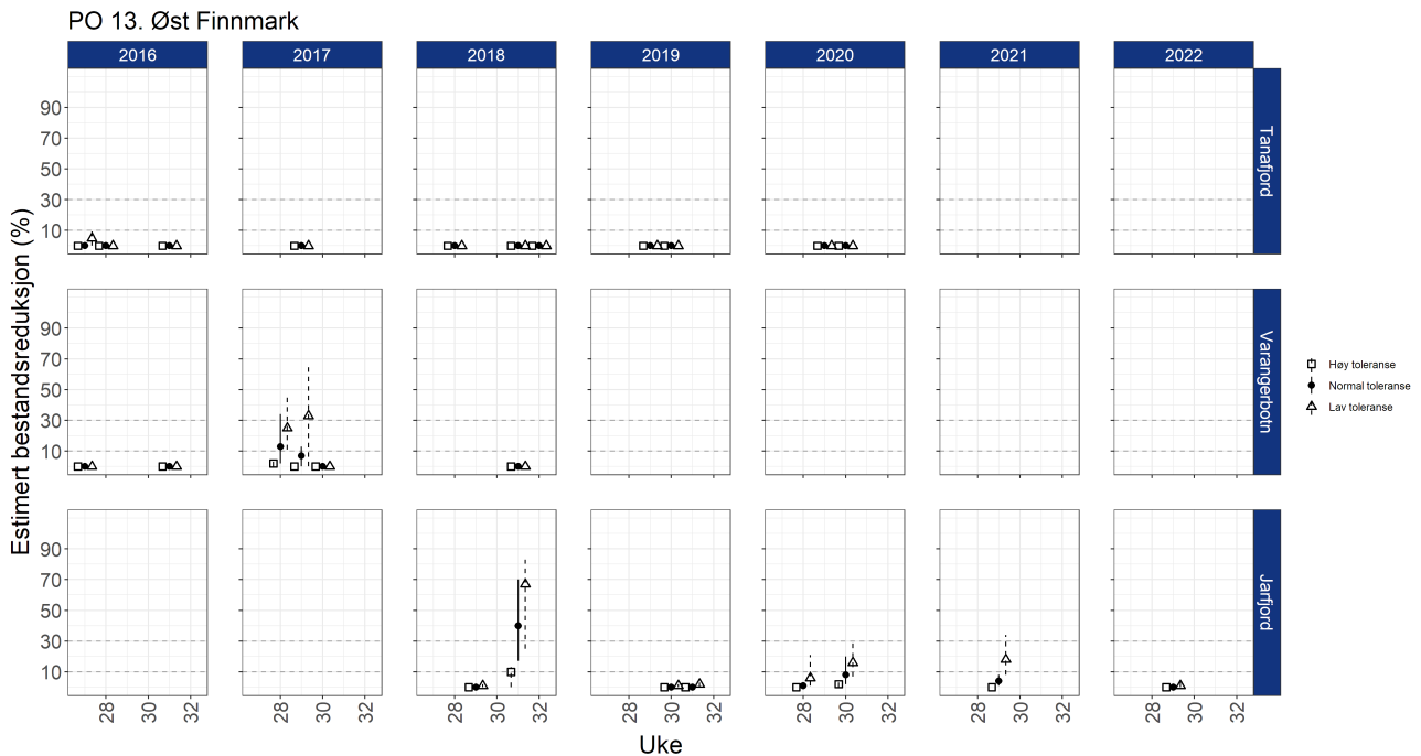
Figur A13. Estimert risiko for dødelighet med konfidensintervaller for sjørøret/sjørøye fanget på stasjonene i PO13 beregnet ved å benytte standard (sirkler), lav (trekanter) eller høy (firkanter) toleransegrenser (Tabell A1). Alle beregningene er basert på sjørøret/sjørøye < 150 g.
