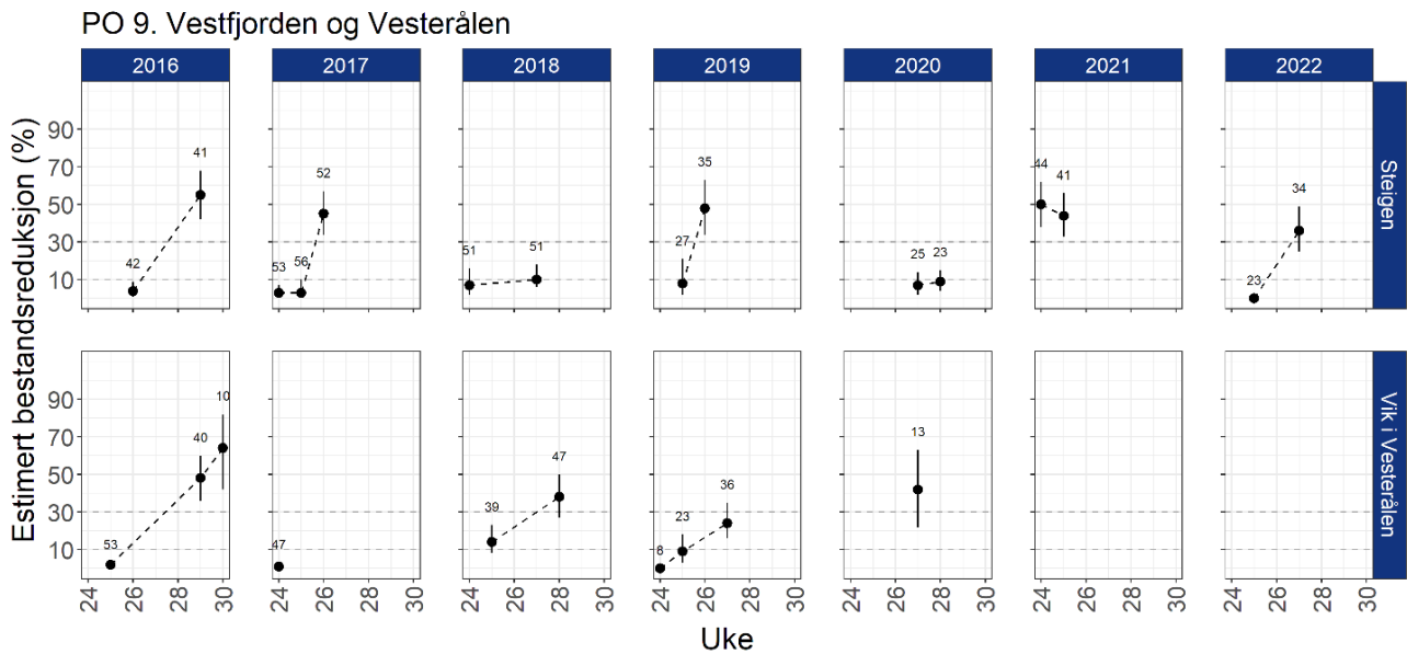
Figur 51. Estimert luseindusert dødelighet på rusefanget sjørrret/sjøørøye med 95% konfidensintervaller. Alle beregningene er basert på all fisk fanget og alle lusestadier.
