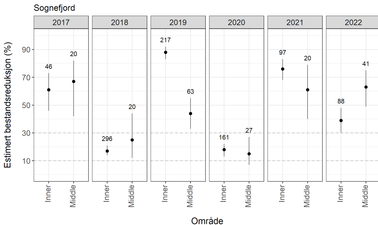
Figur 27. Risiko for lakselusrelatert dødelighet (med konfidensintervaller) på trålfanget vill postsmolt av laks tilordnet hjemmelv. Antall er angitt i figuren. Elvene er gruppert i regioner.
