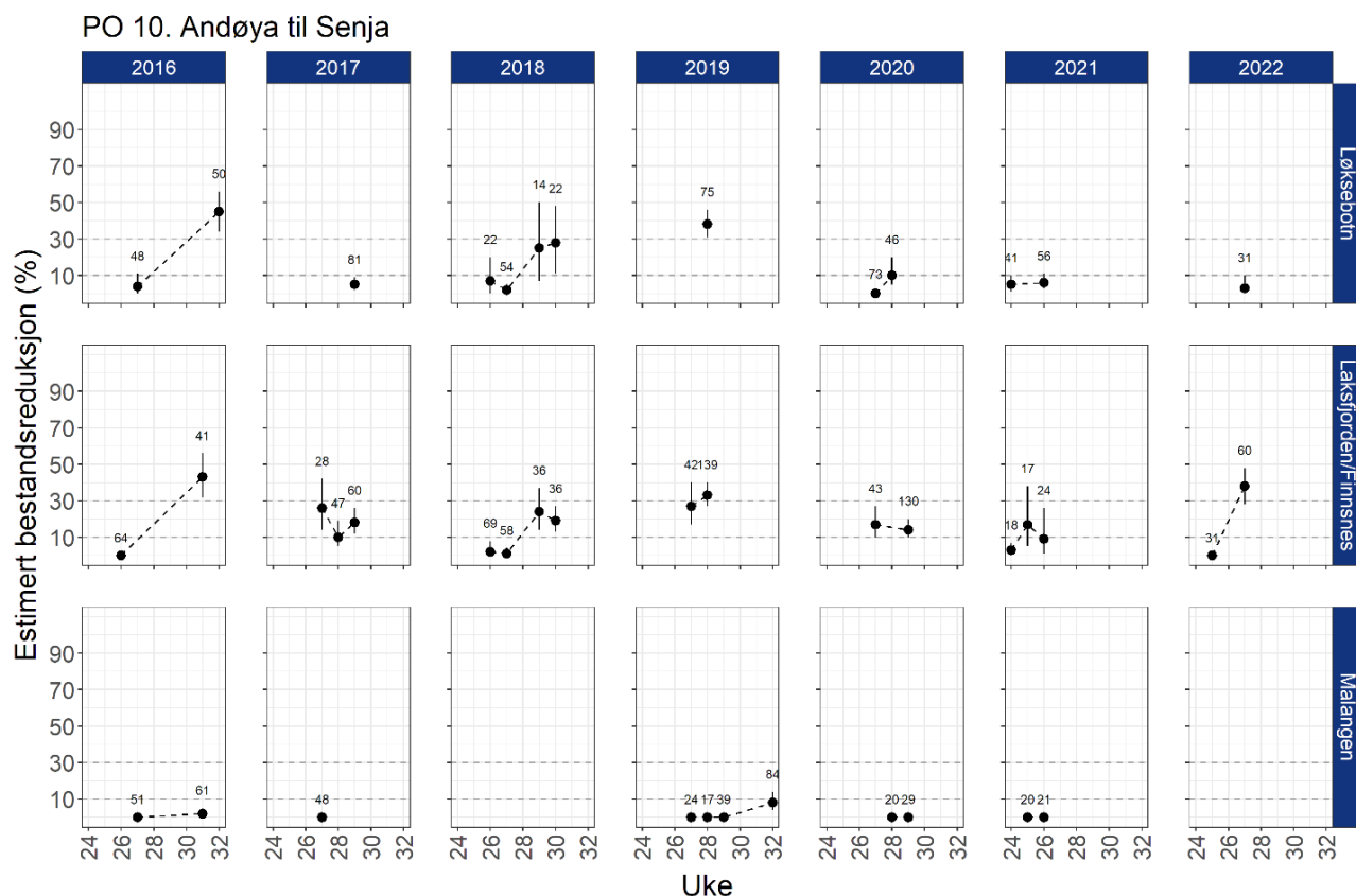
Figur 54. Estimert luseindusert dødelighet på rusefanget sjørret/sjørøye med 95% konfidensintervaller. Alle beregningene er basert på all fisk fanget og alle lusestadier.
