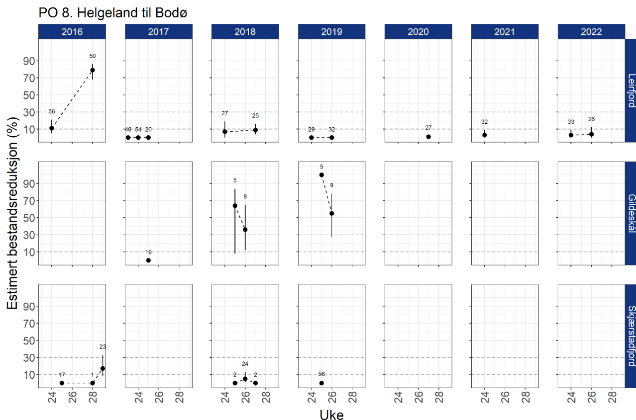
Figur 48. Estimert luseindusert dødelighet på rusefanget sjørrret/sjørøye med 95% konfidensintervaller. Alle beregningene er basert på all fisk fanget og alle lusestadier.
