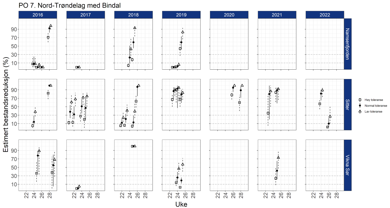
Figur A7. Estimert risiko for dødelighet med konfidensintervaller for sjørøret fanget på stasjonene i PO7 beregnet ved å benytte standard (sirkler), lav (trekanter) eller høy (firkanter) toleransegrenser (Tabell A1). Alle beregningene er basert på sjørøret/sjørøye < 150 g.
