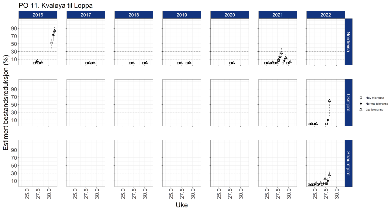
Figur A11. Estimert risiko for dødelighet med konfidensintervaller for sjørøret/sjørøye fanget på stasjonene i PO11 beregnet ved å benytte standard (sirkler), lav (trekanter) eller høy (firkanter) toleransegrenser (Tabell A1). Alle beregningene er basert på sjørøret/sjørøye < 150 g.
