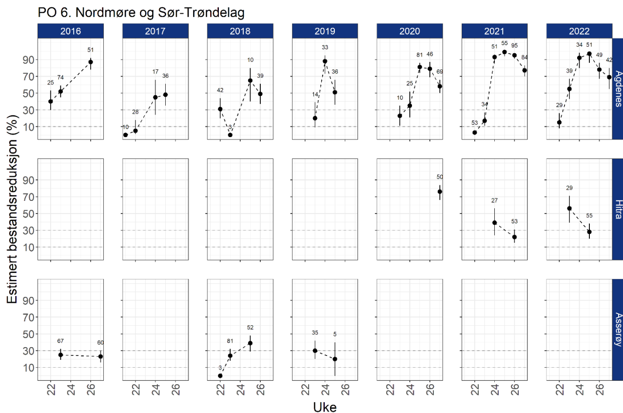
Figur 38. Estimert luseindusert dødelighet på rusefanget sjørrret med 95% konfidensintervaller. Alle beregningene er basert på all fisk fanget og alle lusestadier.
