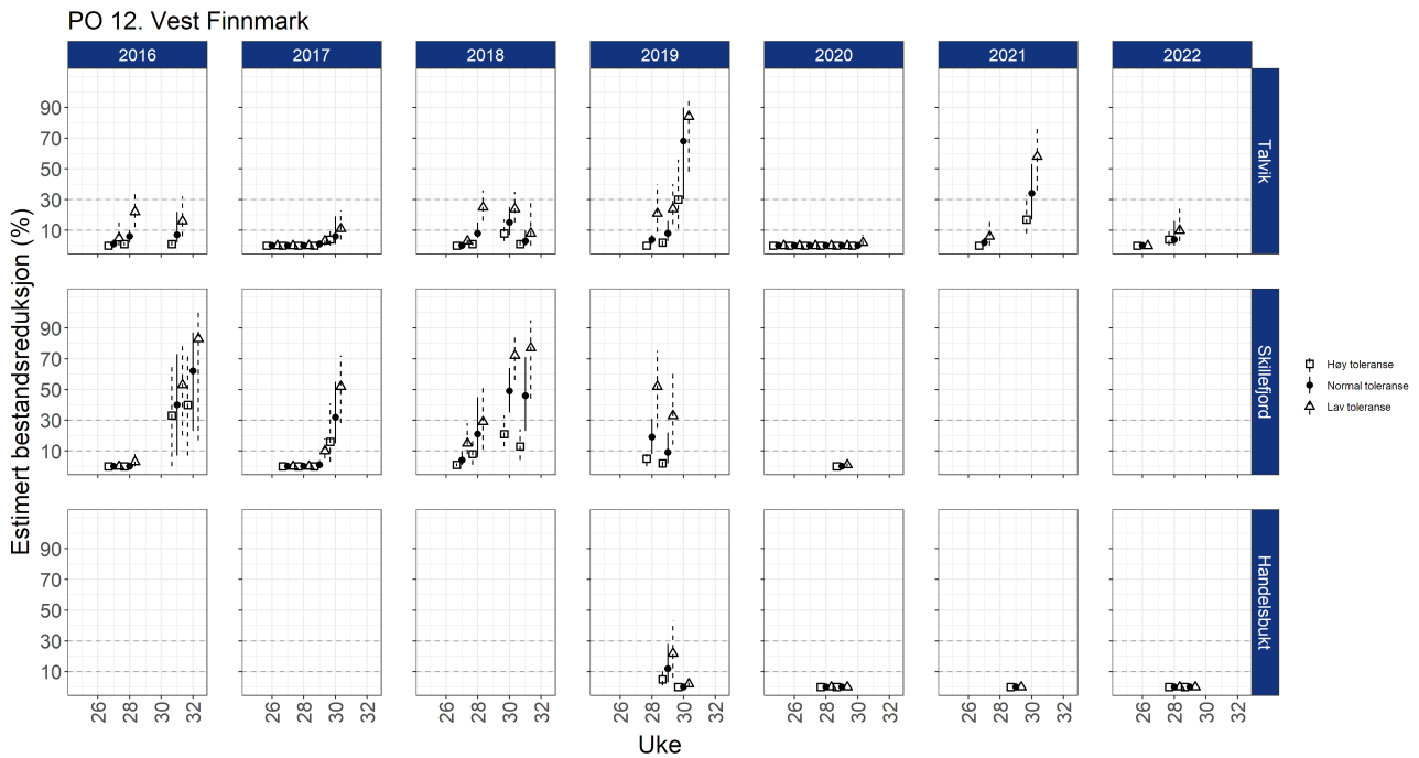
Figur A12. Estimert risiko for dødelighet med konfidensintervaller for sjørøret/sjørøye fanget på stasjonene i PO12 beregnet ved å benytte standard (sirkler), lav (trekanter) eller høy (firkanter) toleransegrenser (Tabell A1). Alle beregningene er basert på sjørøret/sjørøye < 150 g.
