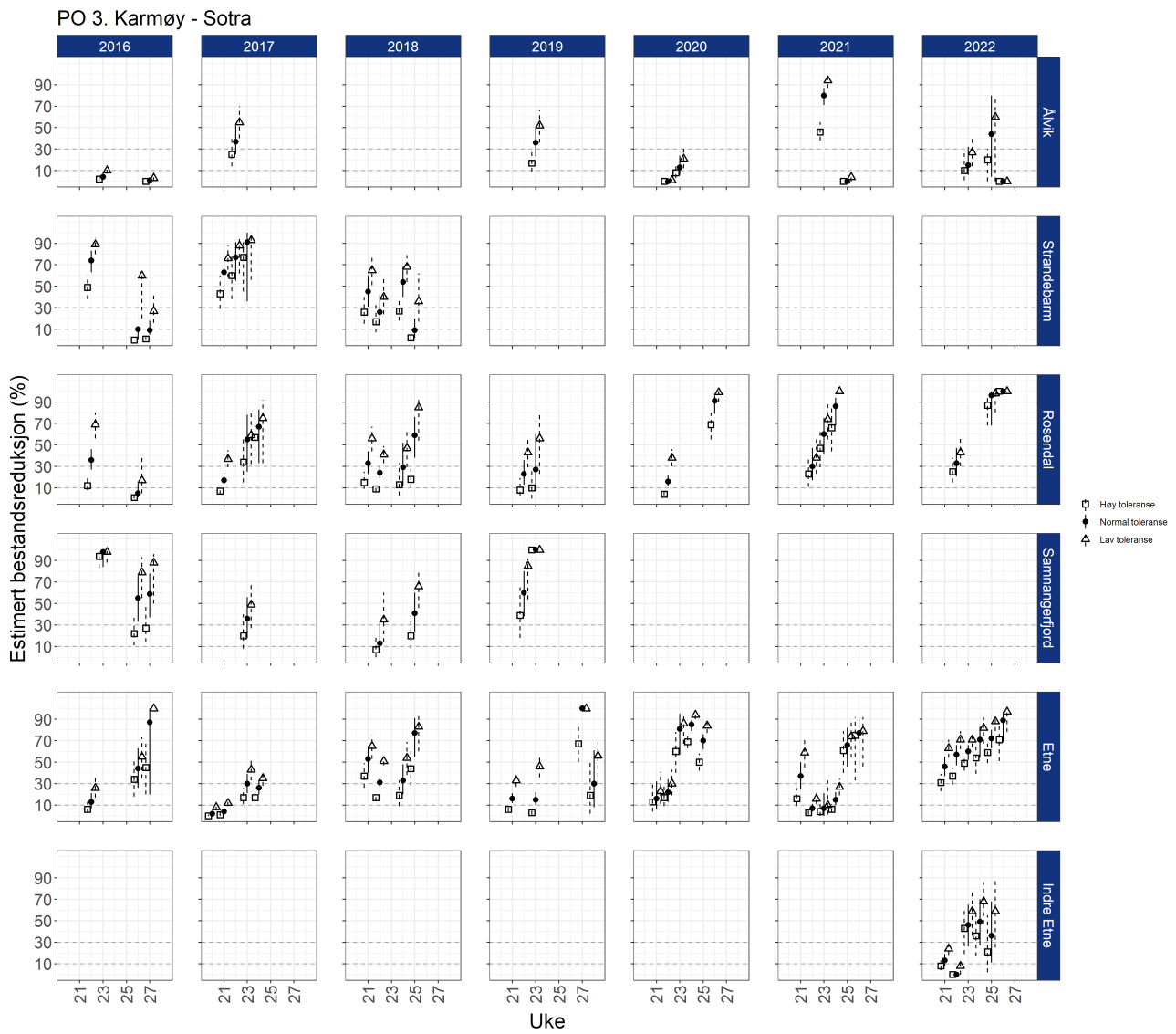
Figur A3. Estimert risiko for dødelighet med konfidensintervaller for sjøørret fanget på stasjonene i PO3 beregnet ved å benytte standard (sirkler), lav (trekanter) eller høy (firkanter) toleransegrenser (Tabell A1). Alle beregningene er basert på sjøørret/sjøørøye < 150 g.
