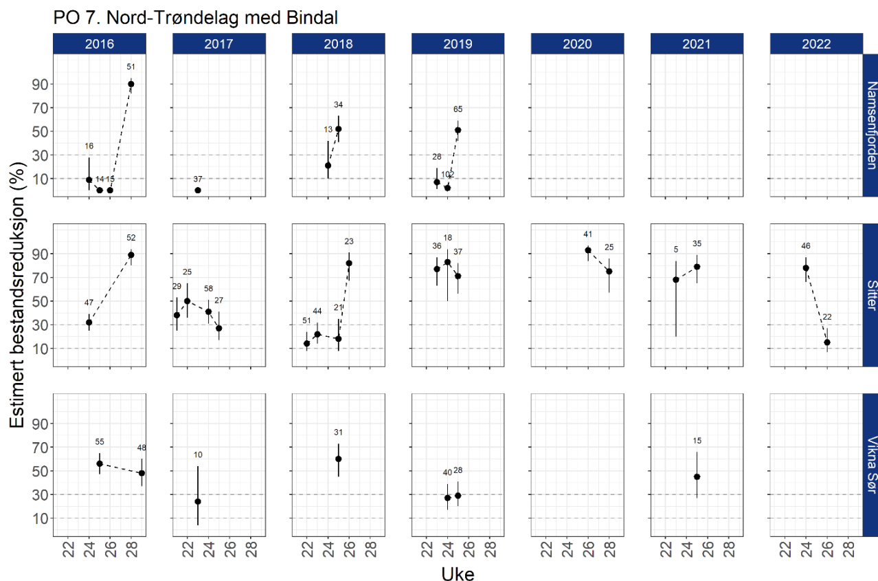
Figur 45. Estimert luseindusert dødelighet på rusefanget sjørrret med 95% konfidensintervaller. Alle beregningene er basert på all fisk fanget og alle lusestadier.
