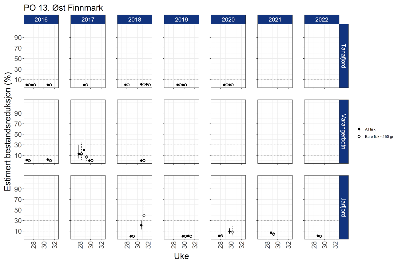
Figur C13: Estimert risiko for dødelighet med konfidensintervaller for sjørøret/sjørøye fanget på stasjonene i PO13 beregnet enten ved å bare inkludere fisk < 150 g, eller all sjørøret/sjørøye fanget.
