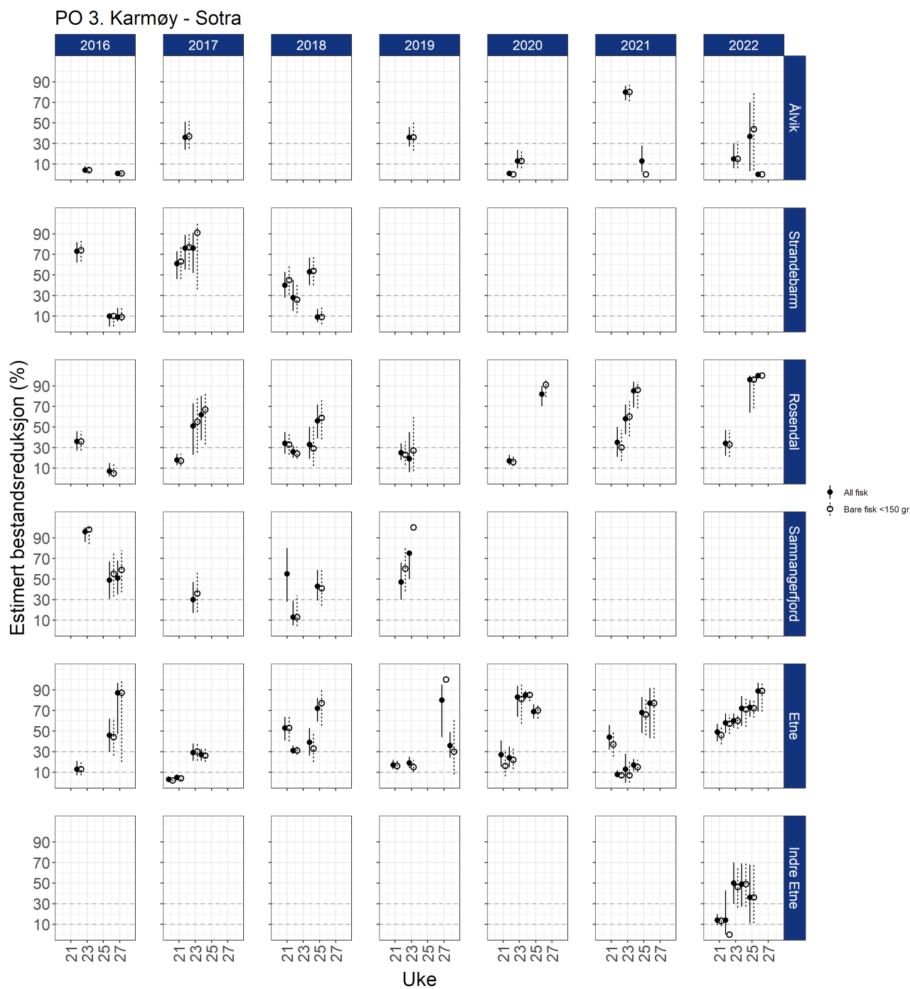
Figur C3: Estimert risiko for dødelighet med konfidensintervaller for sjørøret/sjørøye fanget på stasjonene i PO3 beregnet enten ved å bare inkludere fisk < 150 g, eller all sjørøret/sjørøye fanget.
