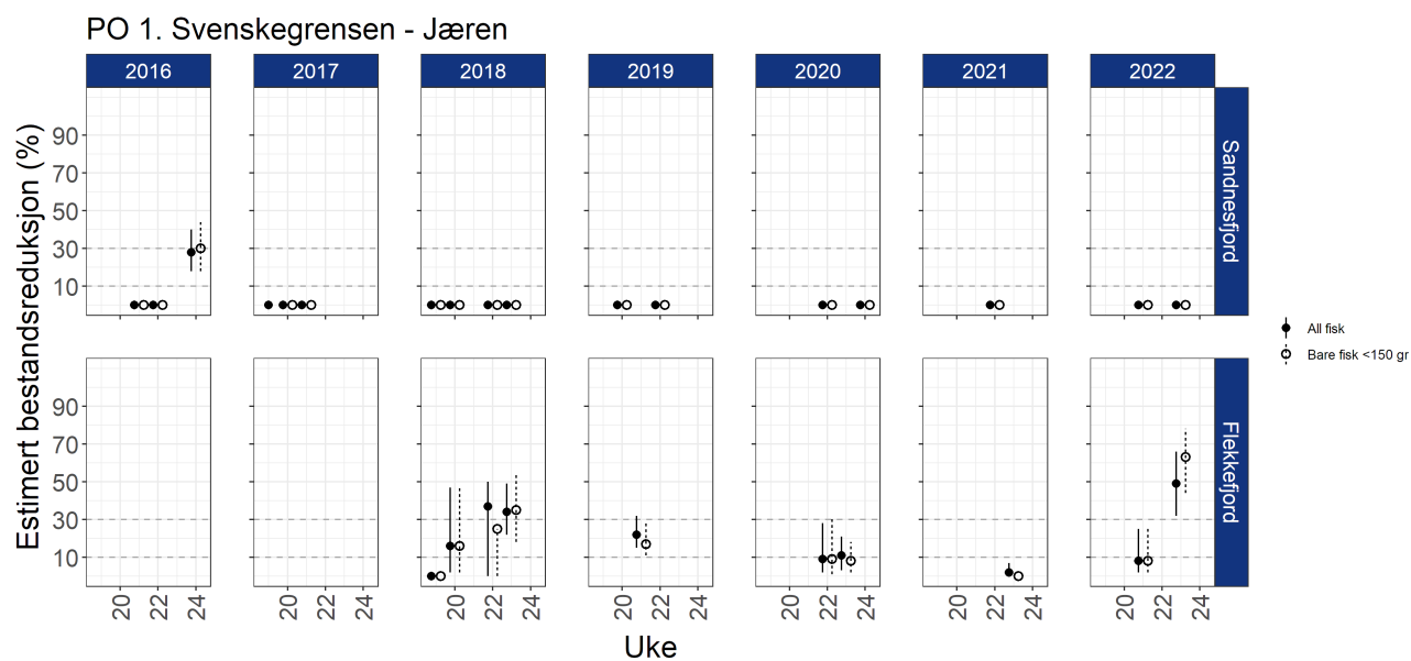
Figur C1: Estimert risiko for dødelighet med konfidensintervaller for sjørørret/sjørøye fanget på stasjonene i PO1 beregnet enten ved å bare inkludere fisk < 150 g, eller all sjørørret/sjørøye fanget.
