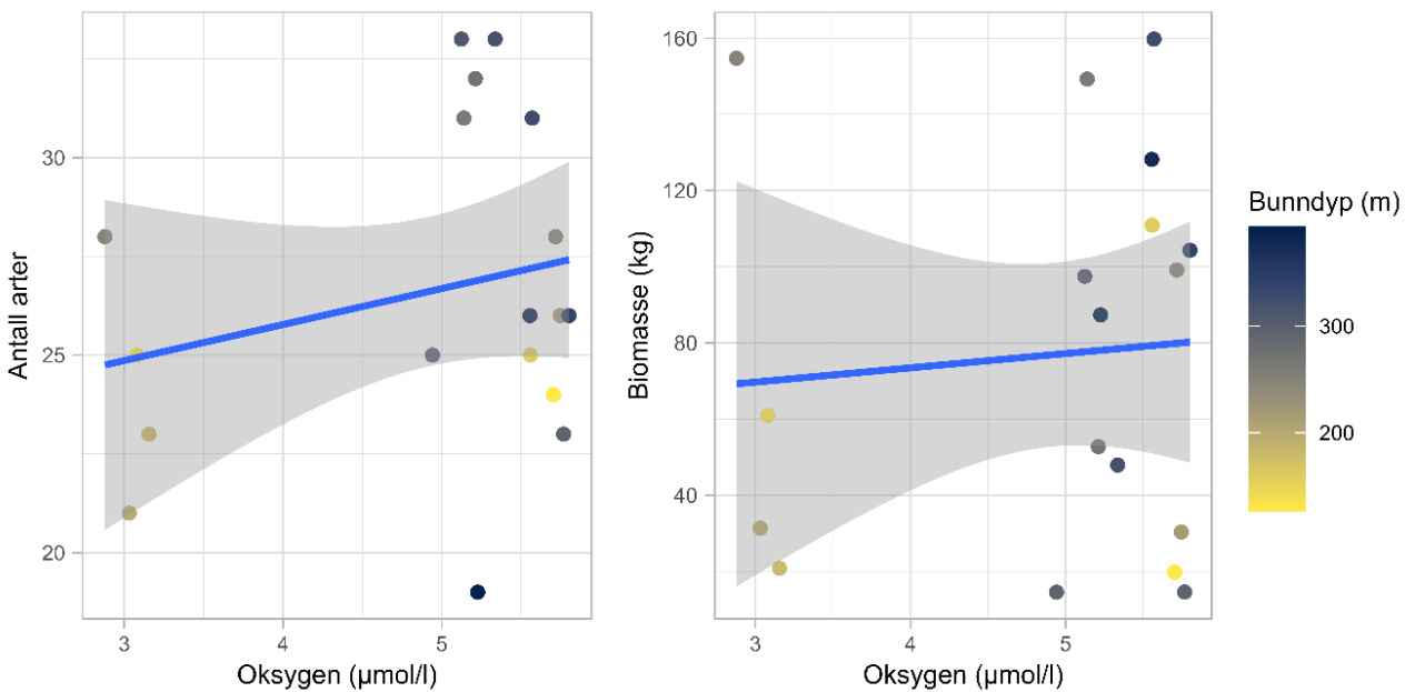
Figur 6.58. Sammenhengen mellom oksygeninnhold og artsdiversitet (venstre) og totalbiomasse (uten kronemaneter, høyre). Fargede punkter representerer observasjoner fra de 18 bunnrålstasjonene, blå linjer og grå områder viser trendlinjen basert på en lineær regresjon (gjennomsnitt og 95 % konfidensintervall). Bunndyp (meter) per trålstasjon er indikert med en fargeskala.
