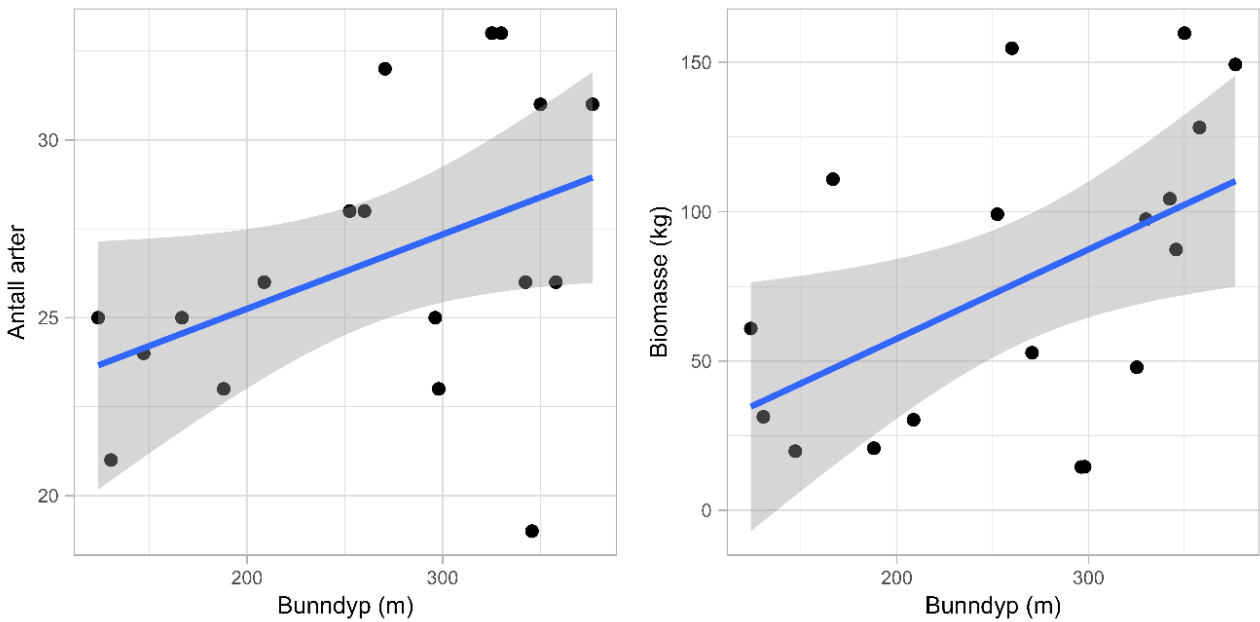
Figur 6.57. Sammenhengen mellom bunndyp (meter) og artsdiversitet (venstre) og totalbiomasse (uten kronemaneter, høyre). Svarte punkter representerer observasjoner fra de 18 bunnrålstasjonene, blå linjer og grå områder viser trendlinjen basert på en lineær regresjon (gjennomsnitt og 95 % konfidensintervall).
