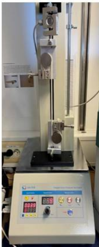
Figur 4.7 Elektrisk strekkcelle med steppermotor, spesifikt laget for testing av strekk og bruddstyrke. Her ble det montert samme tensiometer som på den hydrauliske strekkcellen benyttet i 2021.
