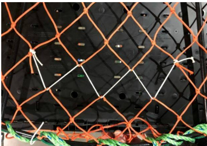
Figur 4.6 Montering av bomullstråd ble utført ved å kutte 6 stolper (3 masker), knytte tråden i ene enden og deretter tre den gjennom maskene og knyte i andre enden. Monteringen tok ca. 1 minutt per teine etter noe trening.
