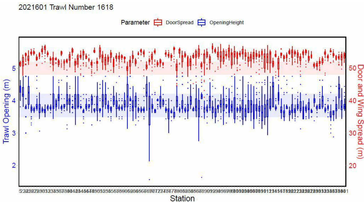
Figur 4.1: Dørspreidning (rød) og trålhøyde (blå) for alle trålhal med Campelen-trål 1618 på reketoktet i 2021. Boksplottene viser median (horisontal linje) med 25 og 75 % kvartiler mens de vertikale linjene viser 1,5 × interkvartil range. De skraverte områdene viser de tidligere tillatte intervallene (3,5–4,2 m for trålhøyde og 48–52 m for dørspreidning).
