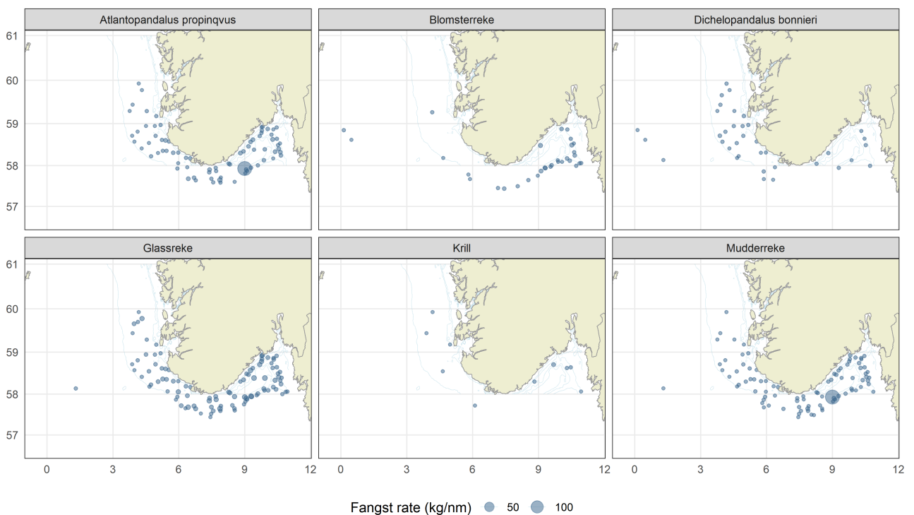
Figur 6.20: Fordeling av Atlantopandalus propinqvus , Pandalus montagui (blomsterreke), Dichelopandalus bonnieri , Pasiphea spp (glassreker), Euphausiacea (krill) og Pontophilus spp (mudderreker) på reketoktet i 2021. Størrelsen på boblene er proporsjonal med fangstraten (kg/nm).
